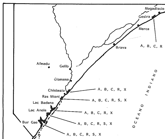
FIG. 1 - Distribuzione e composizione dei mangrovi in Somalia. A = Avicennia marina (Forsk.) Vierh.; B = Bruguiera gymnorrhiza (L.) Lam.; C = Ceriops tagal (Perr.) C.B. Robinson; R = Rhizophora mucronata Lam.; S = Sonneratia alba J.E. Smith; X = Xylocarpus granatum Koenig.
