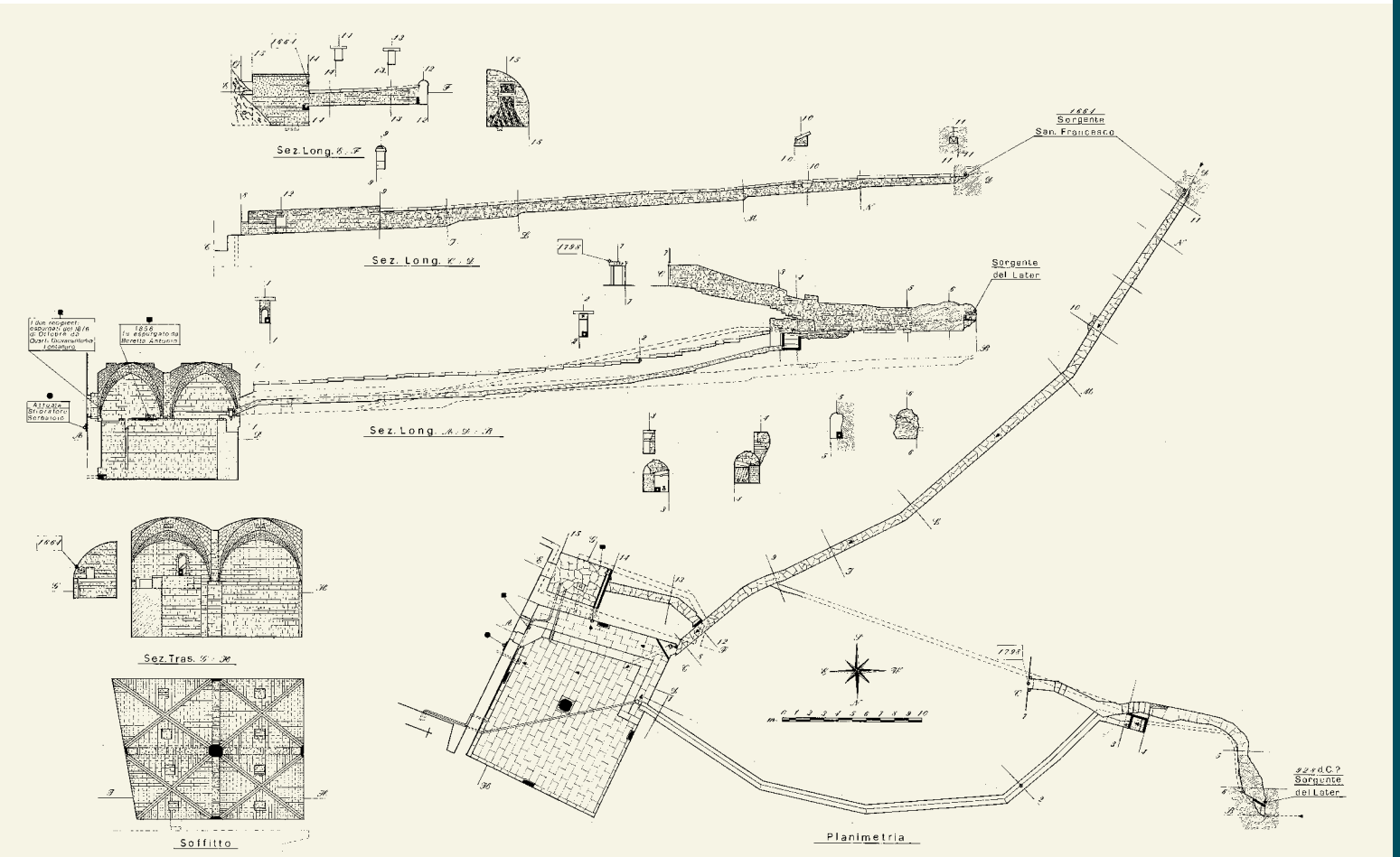
Fontana cisterna del Later (Lantro) – disegno Luca Dell'Olio, Bergamo 1979 (rev. 2014)
