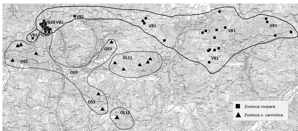
Fig. 1. Distribuzione delle due sottospecie e dei relativi aplotipi.
